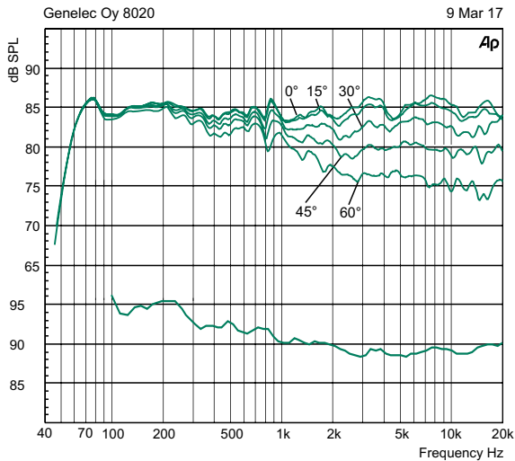
图5 在偏离声轴0°、15°、30°、45°以及60°的功率响应曲线。输入声压级为-20dBu。
