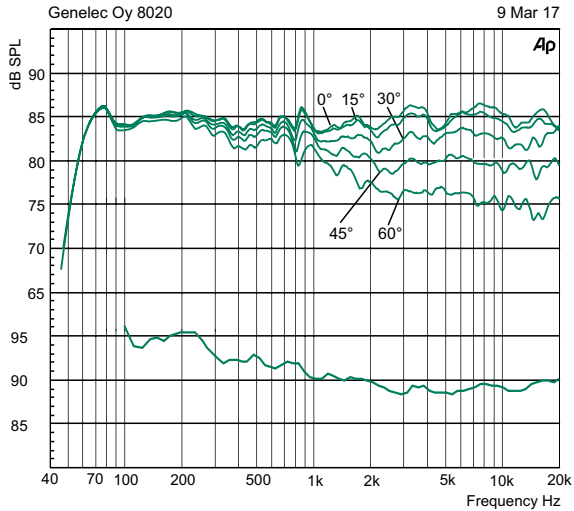
Kuva 5: Ylemmät käyrät esittävät 8020D:n taajuusvasteen eri kulmista mitattuna (kaiutin pystyasennossa, mittauasetäisyys 1 m). Alempi käyrä on kaiuttimen tehovaste.
