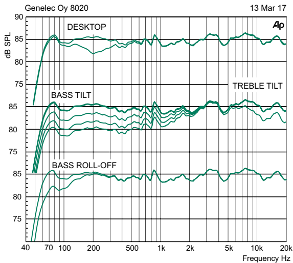
图4 在自由声场下测得8020D受“桌面200Hz控制”，“高频衰减”，“低频衰减”和“低频滚降”控制的频响曲线。
