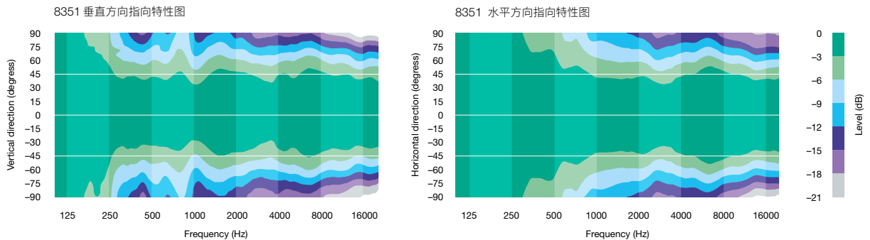
1 图为8351垂直摆放时的指向特性
